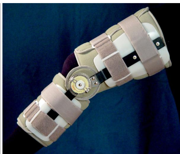
Рис. 4. Ортопедический аппарат с эластичными гильзами, с шарнирами, предусматривающими регулировку угла сгибания
